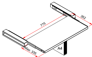
Teleskopboden
