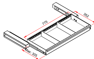
Teleskopschublade
