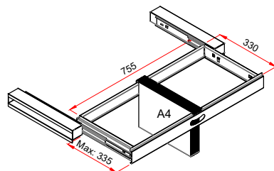
Teleskophängerahmen
