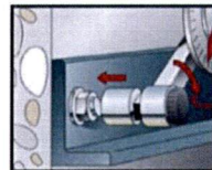
4: Anker mit dem Montage-drehmoment T_{inst} verspreizen
